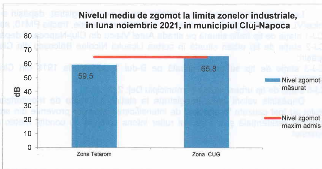
Figura 4.6. Nivelul de zgomot la limita zonelor industriale, în luna noiembrie 2021
