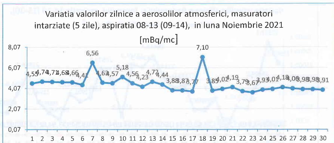
Figura nr. 3.2.3.2 Variația valorilor zilnice a aerosolilor atmosferici, măsurări la 5 zile, aspirația 08-13, în luna Noiembrie 2021
