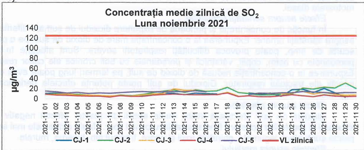
Figura 1.2.1.1. Evoluția concentrației medii zilnice de \text{SO}_2 în județul Cluj în luna noiembrie 2021
