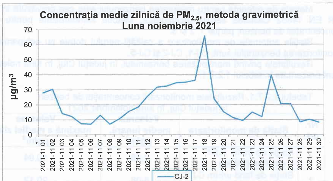
Figura 1.2.5.2. Evoluția concentrației medii zilnice de PM 2,5 , în județul Cluj, în luna noiembrie 2021
