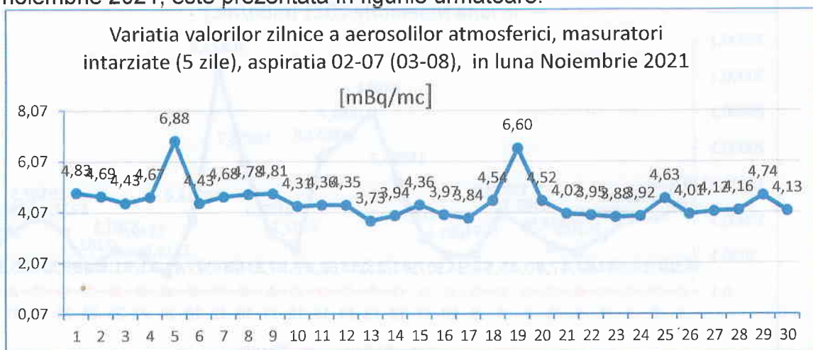
Figura nr. 3.2.3.1 Variația valorilor zilnice a aerosolilor atmosferici, măsurări la 5 zile, aspirația 03-08, în luna Noiembrie 2021
