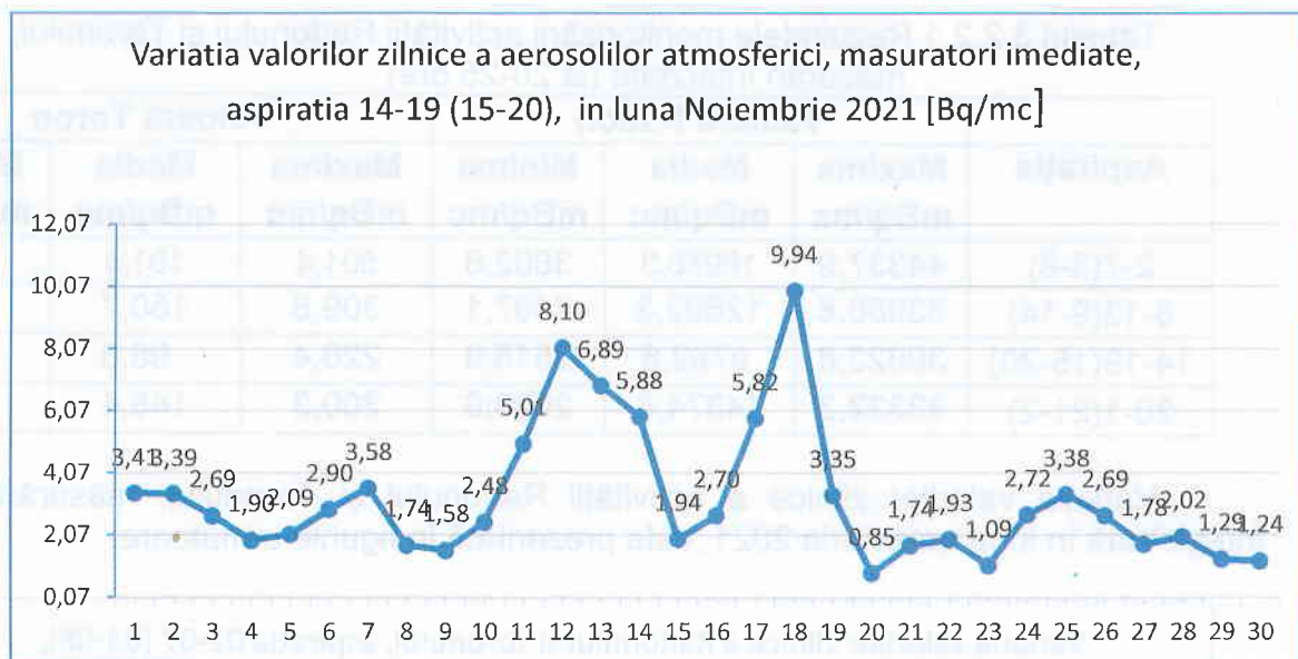
Figura nr. 3.2.1.3 aspirația 14-19
