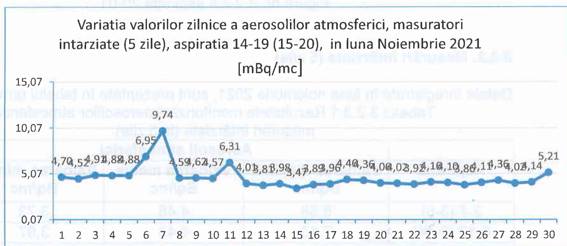
Figura nr. 3.2.3.3 Variația valorilor zilnice a aerosolilor atmosferici, măsurări la 5 zile, aspirația 14-19, în luna Noiembrie 2021
