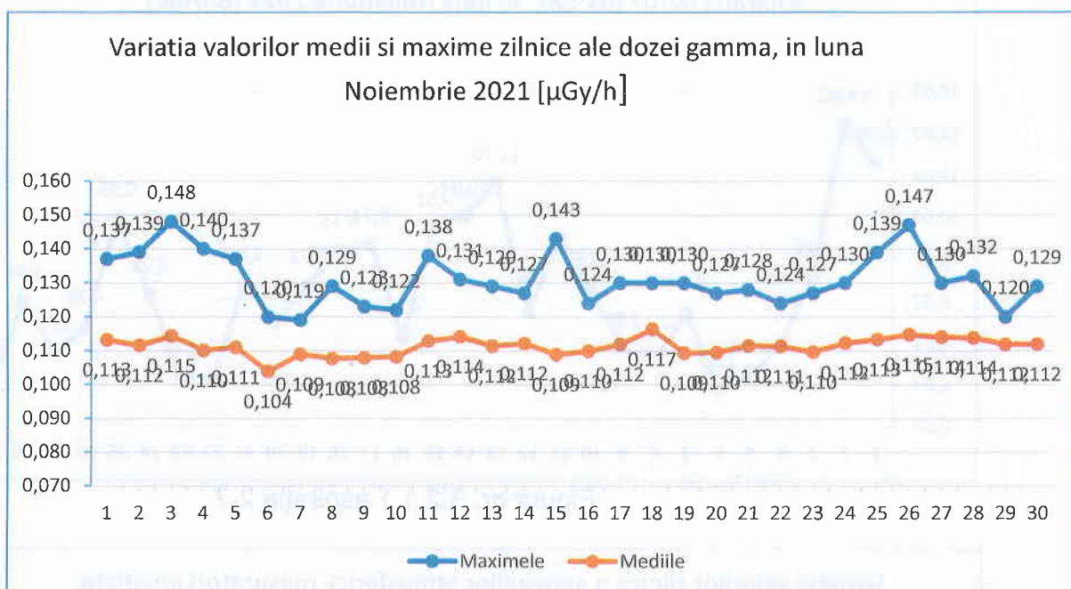
Figura nr. 3.1.1 Variația valorilor medii și maxime zilnice ale debitului dozei gamma în luna noiembrie 2021
