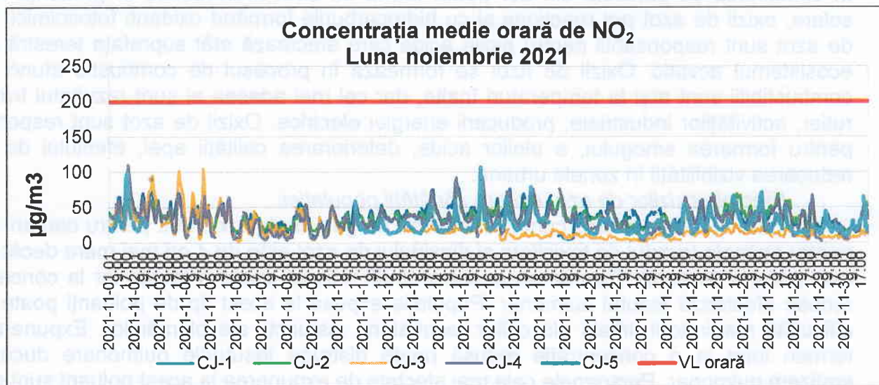
Figura 1.2.2.1. Evoluția concentrațiilor medii orare de \text{NO}_2 în județul Cluj în luna noiembrie 2021
