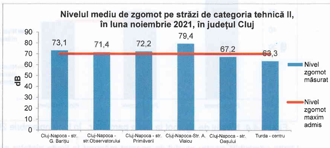
Figura 4.2. Nivelul de zgomot urban pe străzi de categoria II, în județul Cluj, în luna noiembrie 2021
