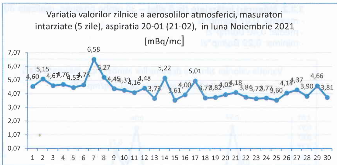
Figura nr. 3.2.3.4 Variația valorilor zilnice a aerosolilor atmosferici, măsurări la 5 zile, aspirația 20-01, în luna Noiembrie 2021
