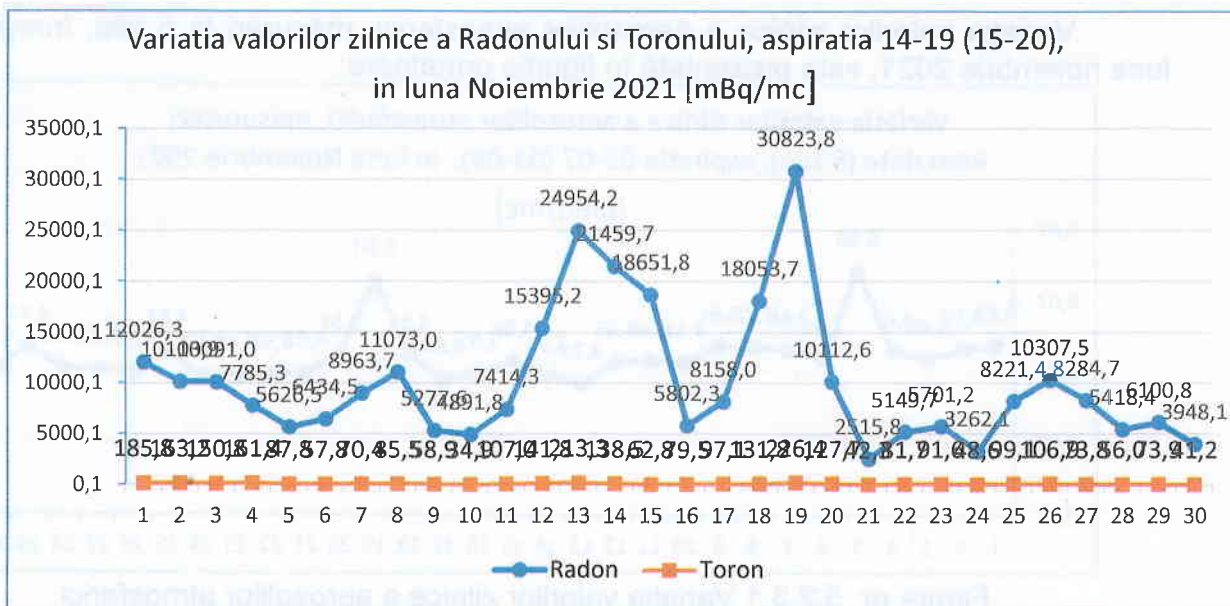
Figura nr. 3.2.2.3 aspirația 14-19
