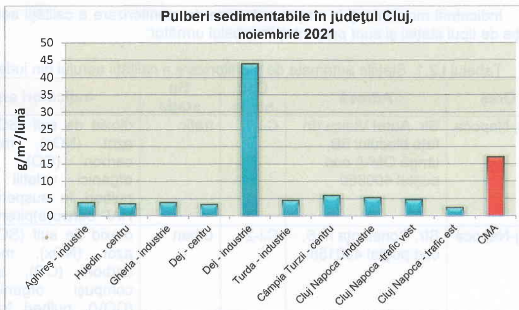
Figura 1.1.4. Evoluția concentrației de pulberi sedimentabile în județul Cluj în luna noiembrie 2021
