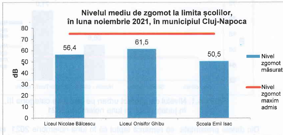
Figura 4.3. Nivelul de zgomot la limita școlilor, în luna noiembrie 2021
