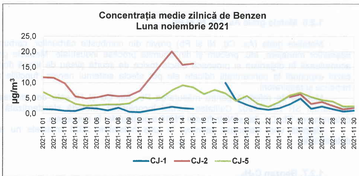
Figura 1.2.7.1. Evoluția concentrației medii zilnice de benzen în județul Cluj, în luna noiembrie 2021
