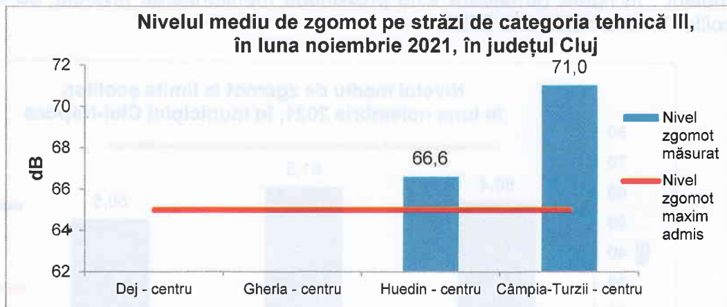
Figura 4.1. Nivelul de zgomot urban pe strazi de categoria III, în județul Cluj, în luna noiembrie 2021
