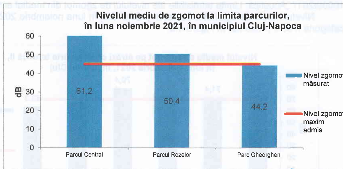
Figura 4.4. Nivelul de zgomot la limita parcurilor, în luna noiembrie 2021
