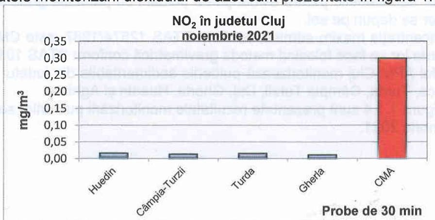
Figura 1.1.2. Evoluția concentrației de dioxid de azot în județul Cluj în luna noiembrie 2021
