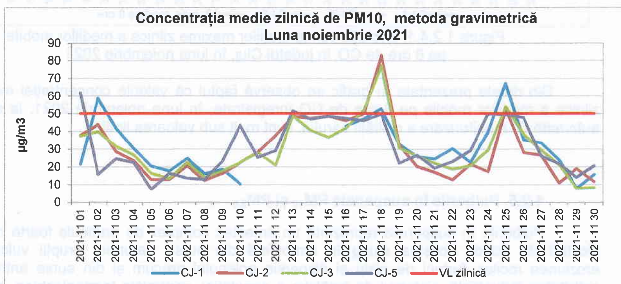
Figura 1.2.5.1. Evoluția concentrației medii zilnice de \text{PM}_{10} , în județul Cluj, în luna noiembrie 2021
