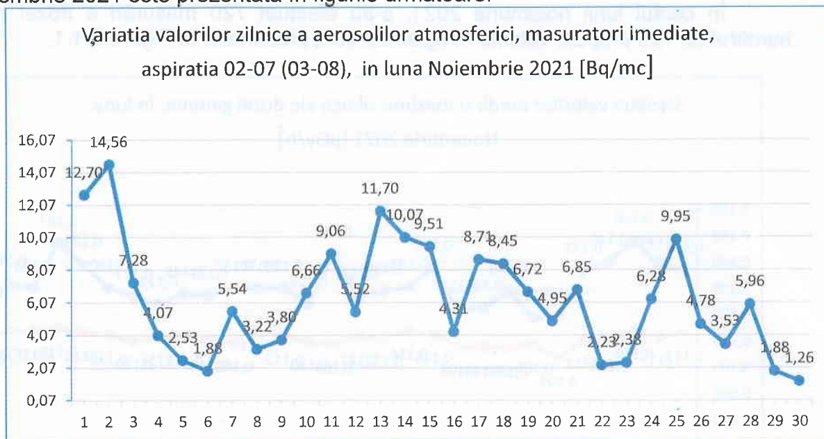
Figura nr. 3.2.1.1 aspirația 2-7
