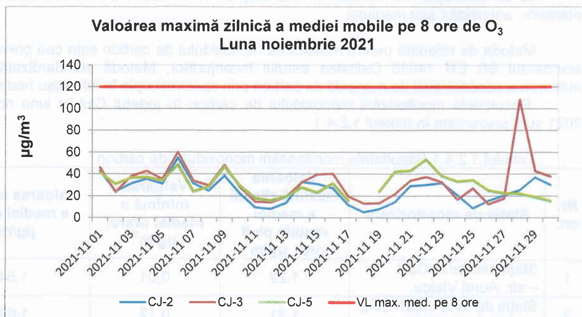
Figura 1.2.3.1. Evoluția maximelor zilnice ale mediilor mobile pe 8 ore de \text{O}_3 , în județul Cluj, în luna noiembrie 2021
