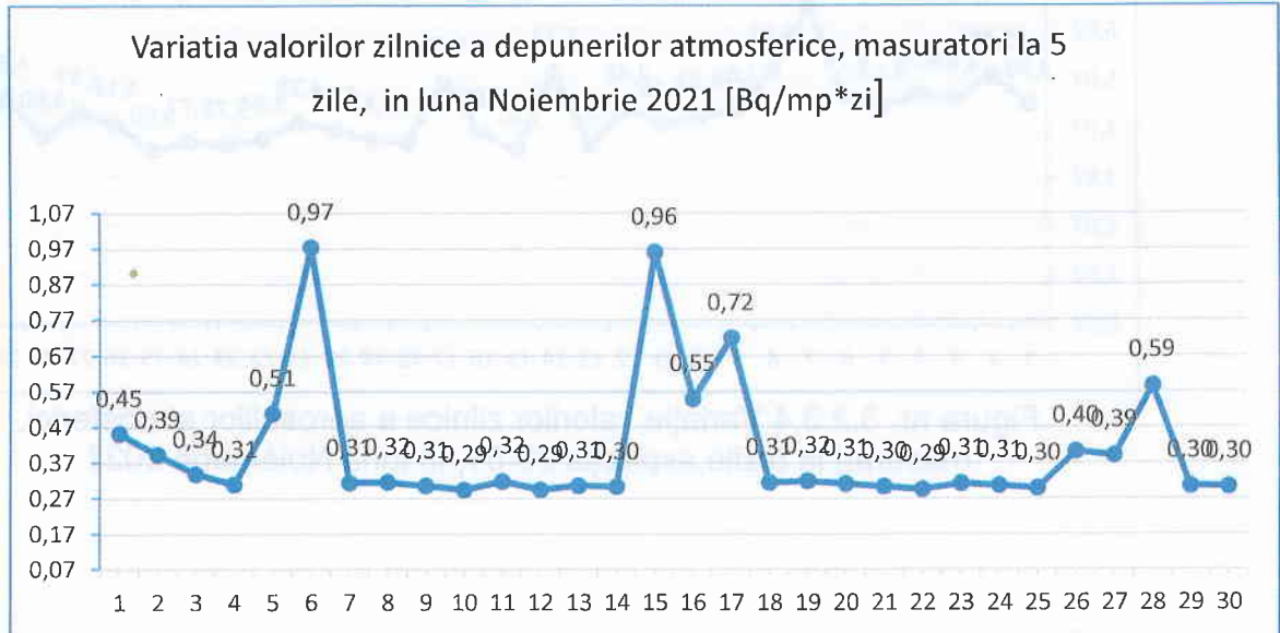
Figura nr. 3.3.2.1 Variația valorilor zilnice a depunerilor atmosferice, măsurări la 5 zile, luna Noiembrie 2021 [Bq/mp*zi]
