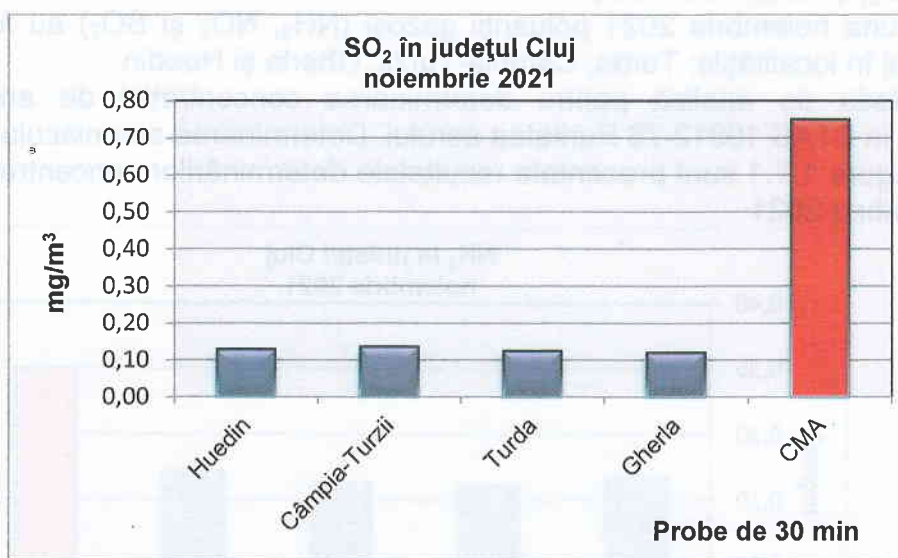
Figura 1.1.3. Evoluția concentrației de dioxid de sulf în județul Cluj în luna noiembrie 2021
