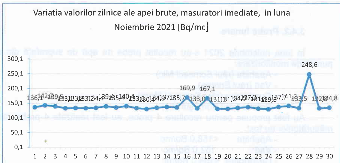
Figura nr. 3.4.1.1.1 Variația valorilor zilnice ale apei brute, măsurări imediate, luna noiembrie 2021
