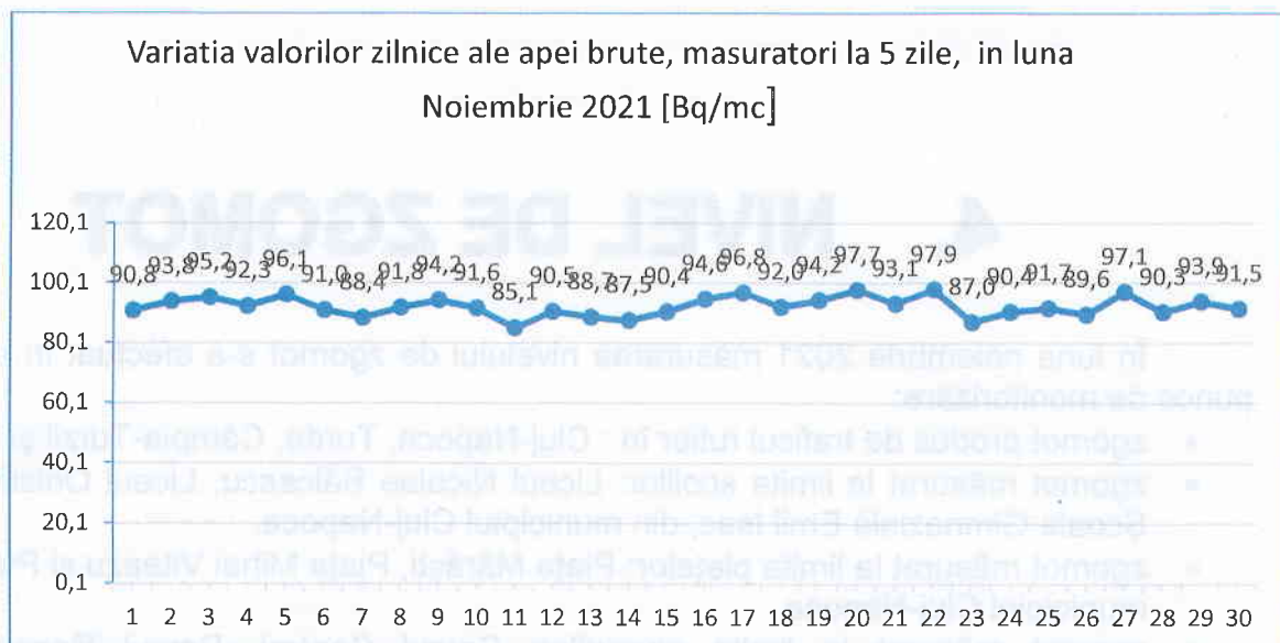
Figura nr. 3.4.1.2.1 Variația valorilor zilnice ale apei brute, măsurări la 5 zile, luna noiembrie 2021
