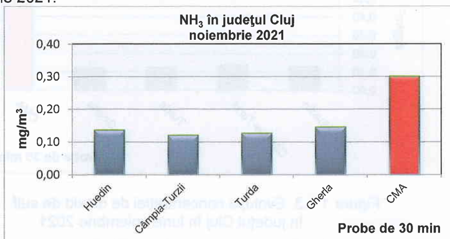
Figura 1.1.1. Evoluția concentrației de amoniac în județul Cluj în luna noiembrie 2021
