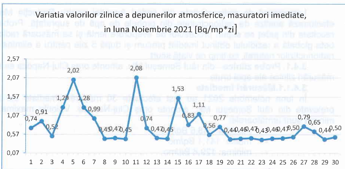
Figura nr. 3.3.1.1 Variația valorilor zilnice a depunerilor atmosferice, măsurări imediate, luna Noiembrie 2021 [Bq/mp*zi]
