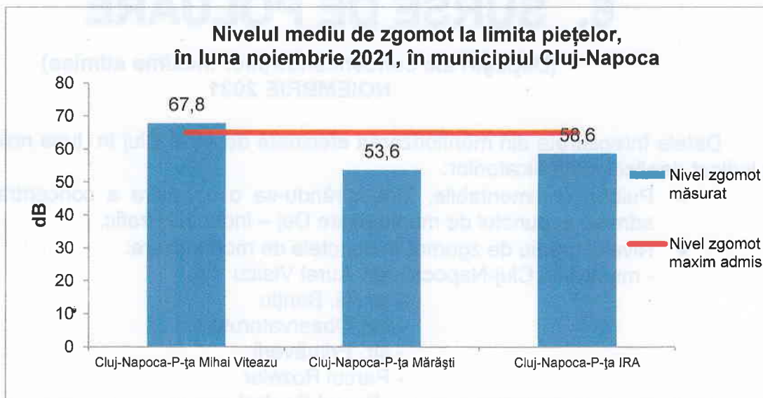
Figura 4.5. Nivelul de zgomot la limita piețelor, în luna noiembrie 2021
