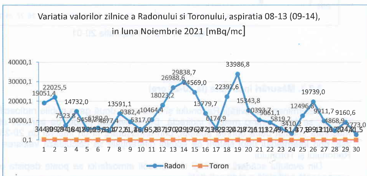
Figura nr. 3.2.2.2 aspirația 8-13
