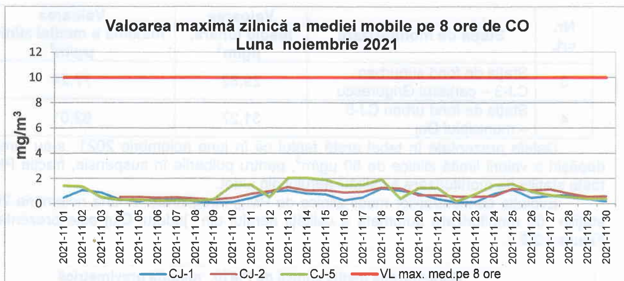
Figura 1.2.4.1. Evoluția concentrațiilor maxime zilnice a mediilor mobile pe 8 ore de CO, în județul Cluj, în luna noiembrie 2021
